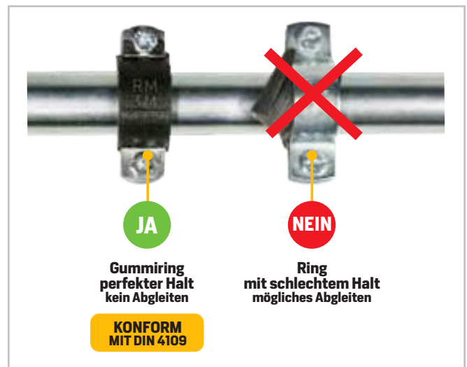
Bild 36 – Gummiring PRATIKO nach DIN 4109 (Unit RM Series 355/G – 351/G – 555/G – 156/G)
