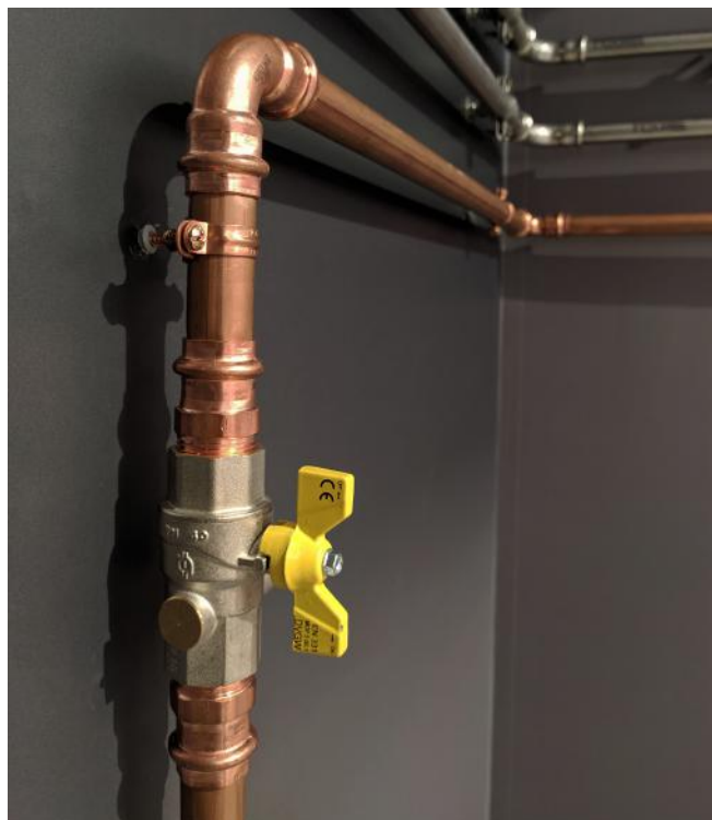
Bild 18 – AesPRES UNIKO GAS – Gasinstallation
