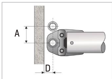
Bild 27 - Mindestabstände und Platzbedarf
