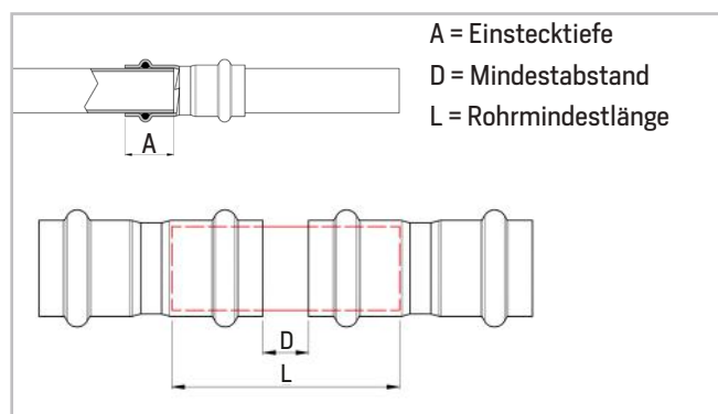
Bild 21 – Einstecktiefe und Mindestabstände
