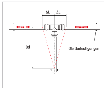
Bild 34 - Dehnungsausgleich (Bd) Abzweig
