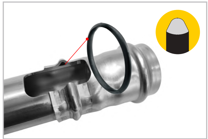
Bild 10 - EPDM Sicherheitsdichtring (ø 15 ÷ 54 mm).
