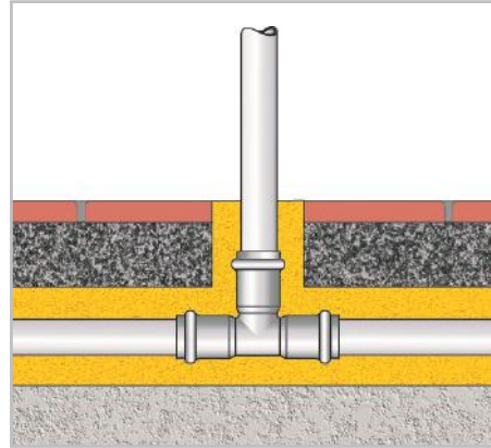
Bild 32b - Schaffung von Ausdehnungsraum
