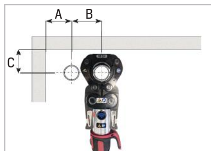
Bild 31 - Mindeststeinbaumaße für Pressschlinge /- Kette
