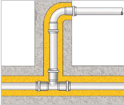
Bild 32a - Schaffung von Ausdehnungsraum
