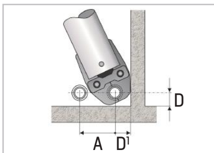
Bild 28 - Mindestabstände und Platzbedarf
