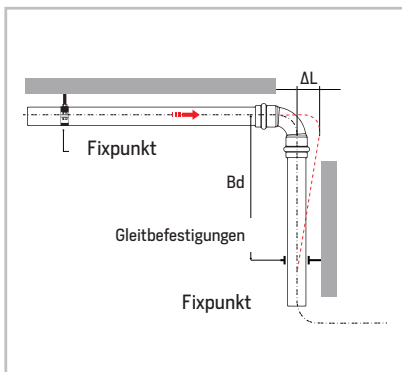
Bild 33 - Dehnungsausgleich (Bd) Rohrschenkel
