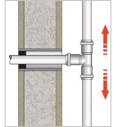
Bild 32c - Schaffung von Ausdehnungsraum
