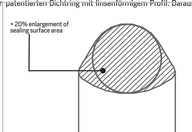
Bild 9 – Dichtringprofil
