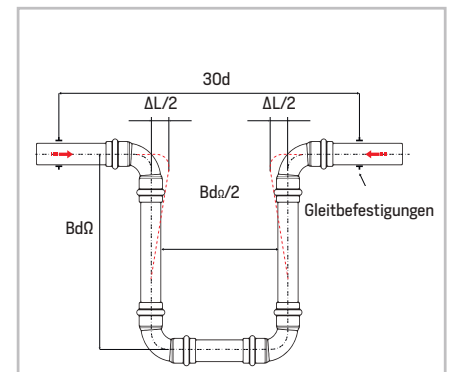
Bild 35 - U-Rohrbogen Bd\Omega = Bd / 1,8
